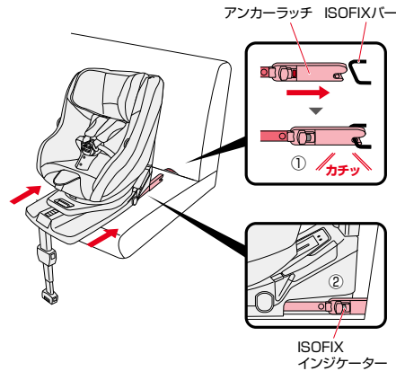
アンカーラッチ ISOFIXバー
