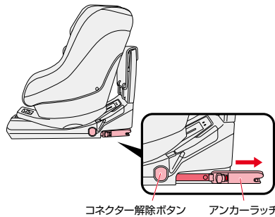
コネクター解除ボタン アンカーラッチ
